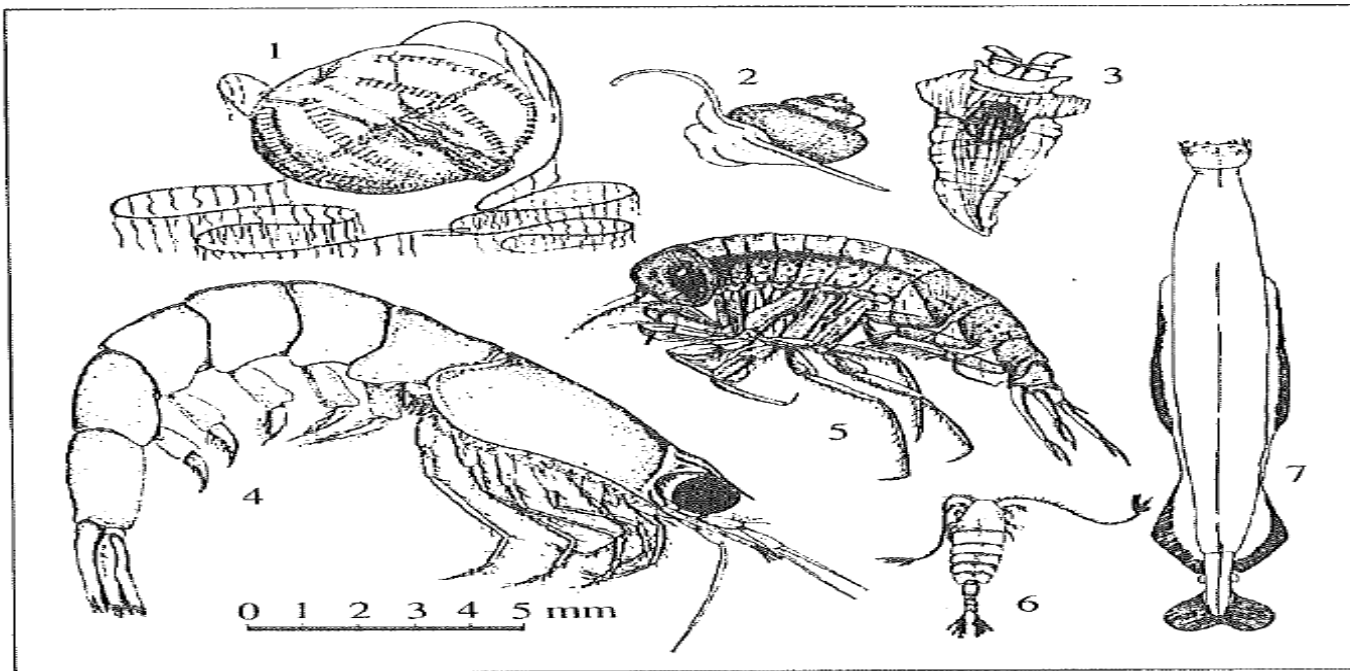
図 8-4 大型動物プランクトンの例 (LeBrasseur and Fulton, 1967)
