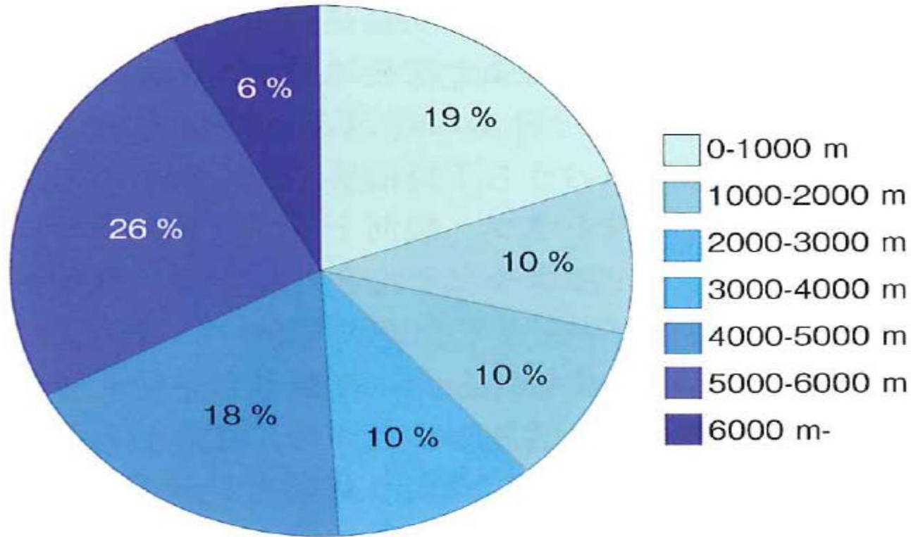
Fig. 1.1. 日本の排他的経済水域内における水深帯の面積比. 松沢(2005)を改変. Areal ratio of each 1000 m depth zone in the Japanese EEZ. Modified from Matsuzawa (2005).
