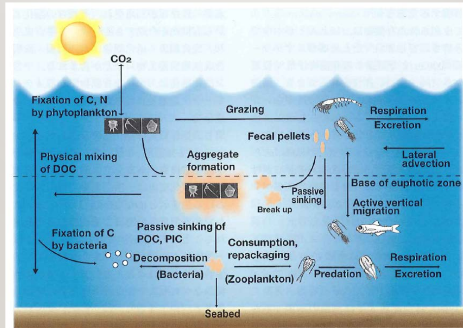
Fig. 2.14. 生物ポンプのダイアグラム. De la Rocha (2006)を改変. Diagram of the biological pump. Modified from De la Rocha (2006).
